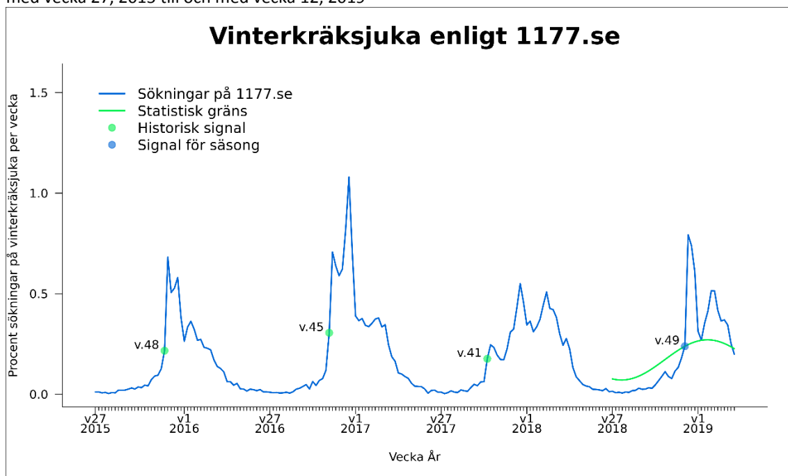
Figur 3. Andelen sökningar på ordet vinterkräksjuka på 1177 Vårdguidens webbplats 1177.se, från och med vecka 27, 2015 till och med vecka 12, 2019
